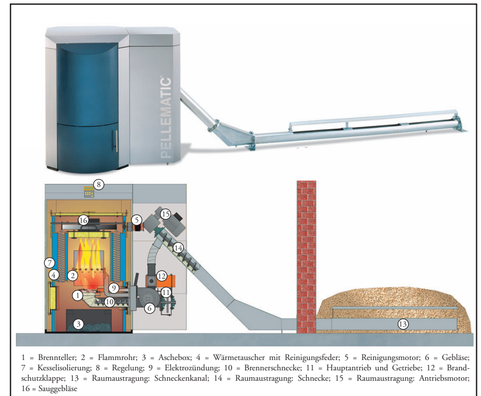
Abb. 5: Beispiel einer Pellet-Zentralheizung mit vollautomatischer Schneckenförderung aus dem benachbarten Lageraum. Die Kosten für eine Zentralheizung variieren je nach Leistung und Komfort zwischen 7 000 € (bis 15 kW) und 13 500 € (bis 45 kW) (Skizze und Bild: ÖkoFEN, Lembach Österreich).
