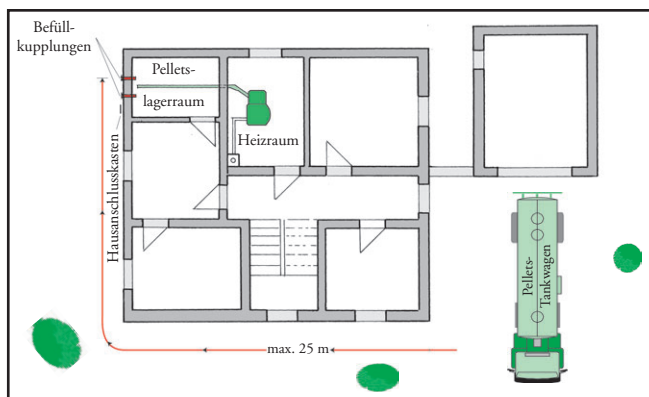
Abb. 11: Beispiel für die Lage des Heizungs- und Pellets-lager-raumes (Skizze: ÖkoFEN, Lembach Österreich).
