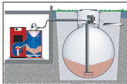
Abb. 12: Beispiel für einen Pellets-lagertank außerhalb des Hauses. Die Pelletsförderung erfolgt durch Saugaustragung (Quelle: Nau GmbH, Moosburg-Pffrombach).
