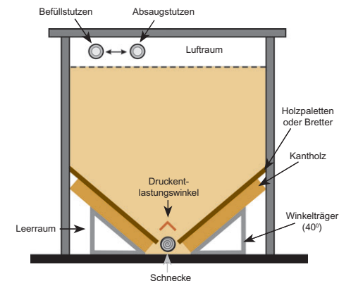
Abb. 13: Schnitt eines Pellets-lager-raumes. Durch den Einbau eines schrägen Zwischenbodens wird die Menge der nicht durch die Förderschnecke austragbaren Pellets verringert. Durch diese Zwischenböden und aufgrund des Luft-raumes, in dem sich die Befüll- und Absaugstutzen befinden, können nur ca. 2/3 des Lagerraumvolumens tatsächlich für die Lagerung der Pellets genutzt werden (Skizze nach ÖkoFEN, Lembach Österreich).
